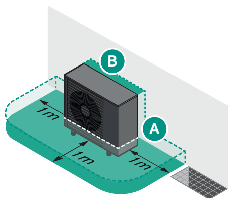
vægmontering
