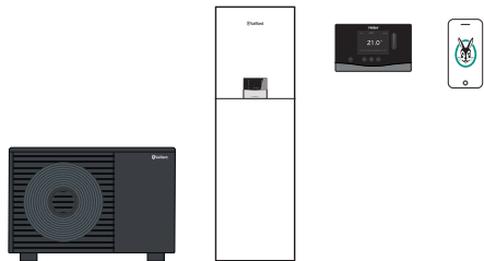
aroTHERM pro luft til vand varmepumpe, unitTOWER hydraulisk tårn, System-automatik sensoCOMFORT, styring via myVaillant-appen
