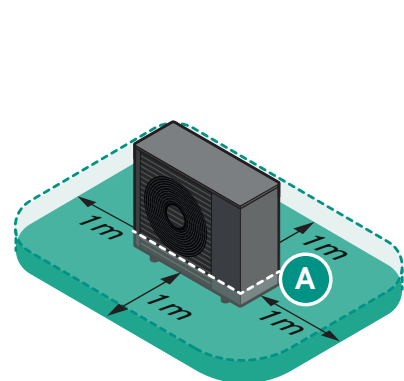
fritstående installation
